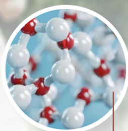
D-манноза
